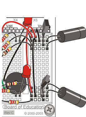
IR pairs close-up
